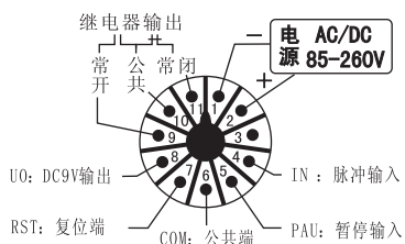
HB48圆端子接线图
