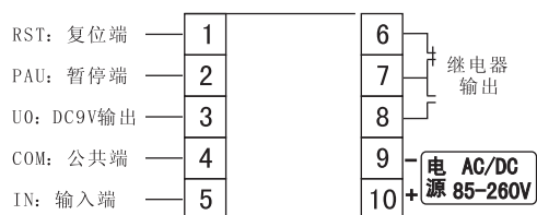
HB48方端子接线图
