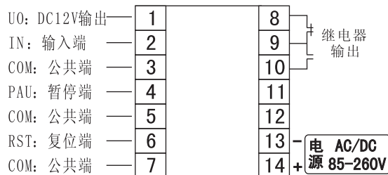
HB72 接线图
